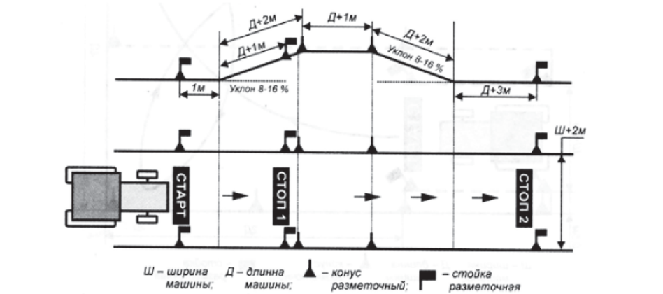
Рис. 7. Остановка и трогание на подъеме
