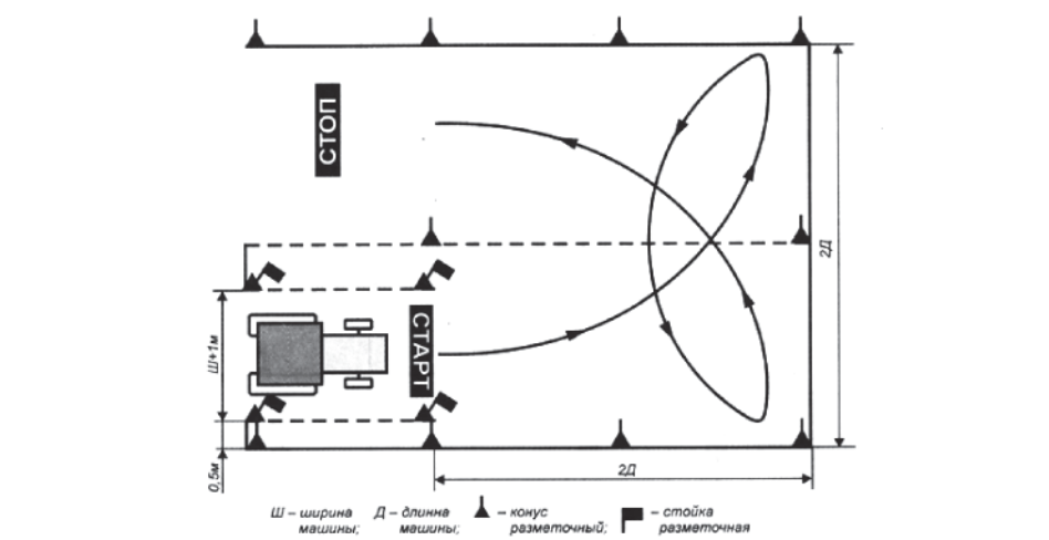
Рис. 8. Разворот, маневрирование в ограниченном пространстве
