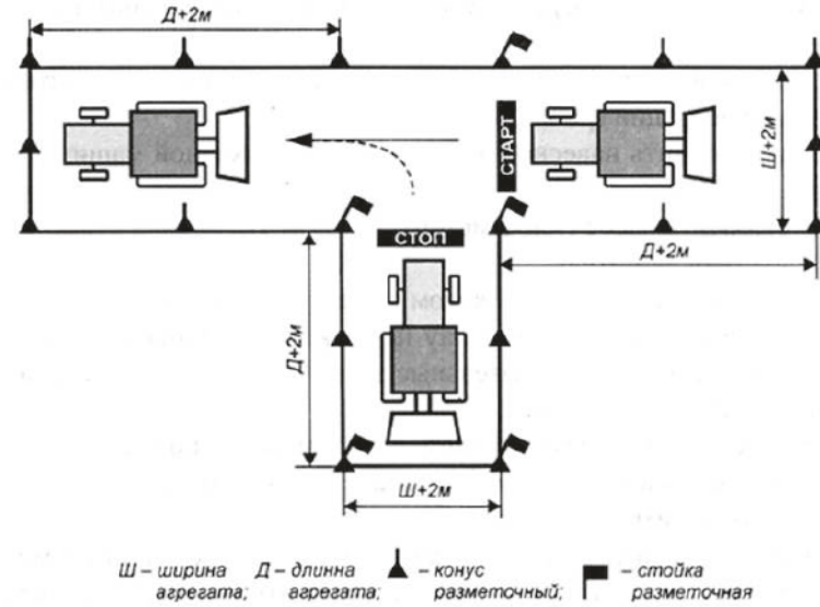
Рис. 12. Агрегатирование с навесной машиной или прицепом
