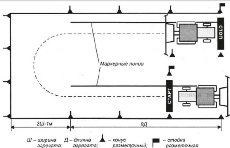
Рис. 15. Движение по маркерной или «провешенной» линии
