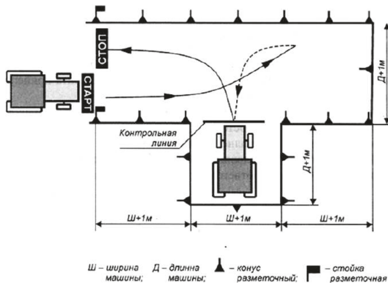
Рис. 9. Постановка самоходной машины в «бокс» задним ходом
