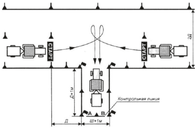
Рис. 10. Движение задним ходом, въезд в «бокс» в агрегате с прицепом
