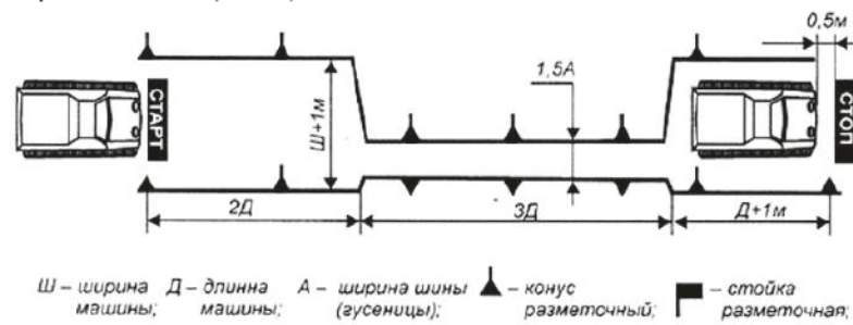
Рис. 13. Колейная доска:
