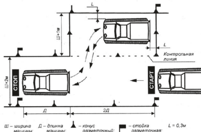
Рис. 18. Парковка СМ задним ходом и выезд с парковочного места, параллельная парковка
