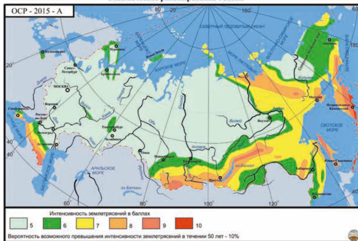
Сейсмическое районирование России
