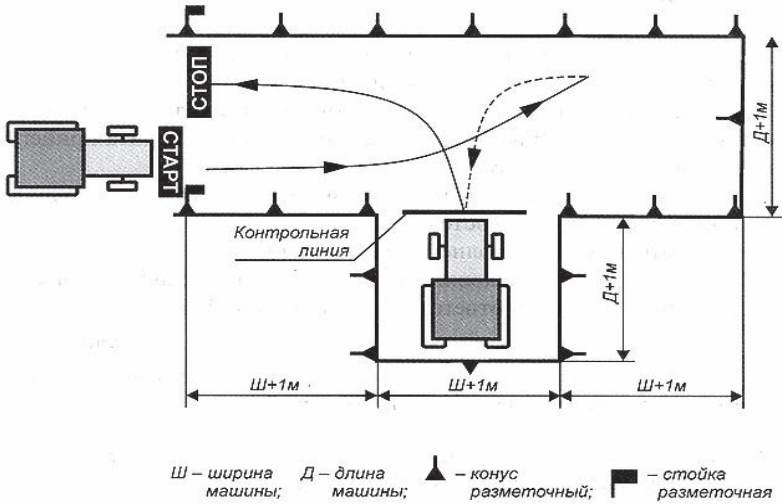
Рис. 6. Постановка самоходной машины в бокс задним ходом
