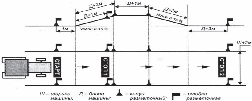
Рис. 4. Остановка и трогание на подъеме
