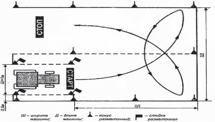
Рис. 5. Разворот, маневрирование в ограниченном пространстве
