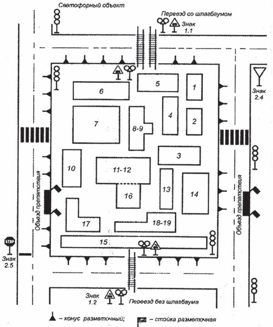
Рис. 1. Схема площадки для проведения практического экзамена
