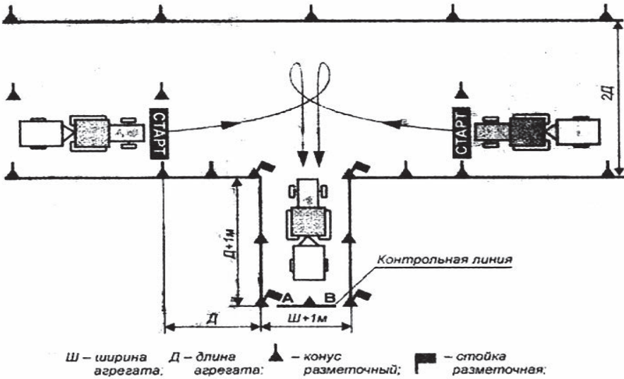
Рис. 7. Движение задним ходом, въезд в бокс в агрегате с прицепом
