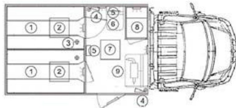
Схема автозака: 1. Общая камера. 2. Аварийный люк. 3. Вентиляционные отверстия. 4. Огнетушитель. 5. Аптечка. 6. Откидной люк. 7. Аварийно-вентиляционный люк; 8. Одиночная камера с лавкой. 9. Отопитель.
