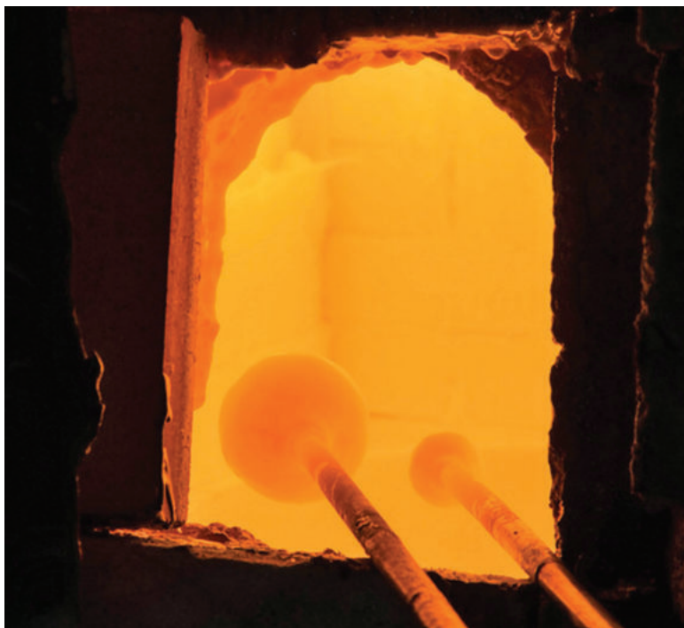
Варка хрусталя в печи.
